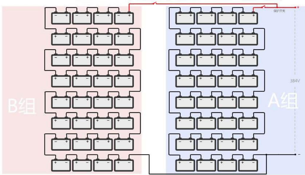
30KVA-100KVA 2 组并接接线示意图
